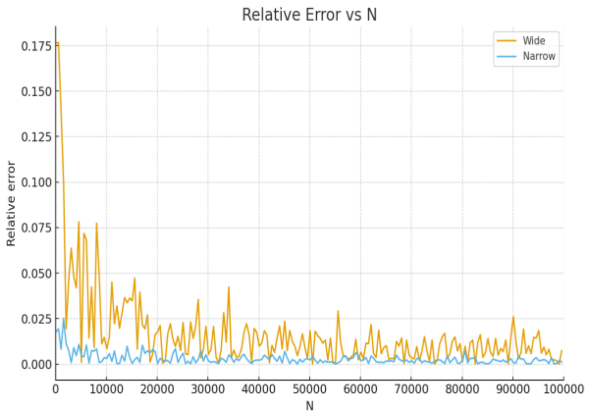
График 2: Относительная ошибка
