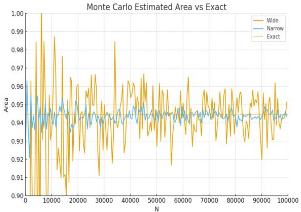
График 1: Приближённая площадь
